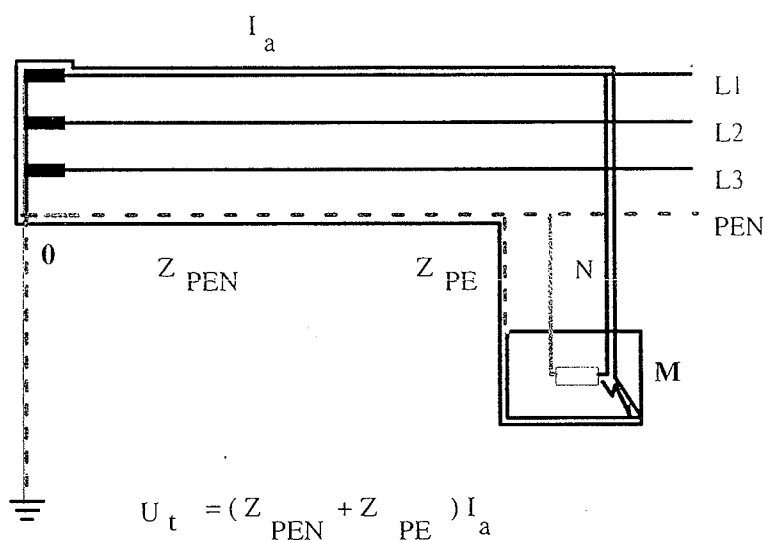
KUVA 41.9. Yksinkertaistettu kuva TN-järjestelmästä, josta käy ilmi TN-järjestelmän suojausperiaate. Vaihejohtimen ja jännitteelle alttiin osan (M) välisessä viassa syntyy vikavirta I_a vikavirtapiiriin.
