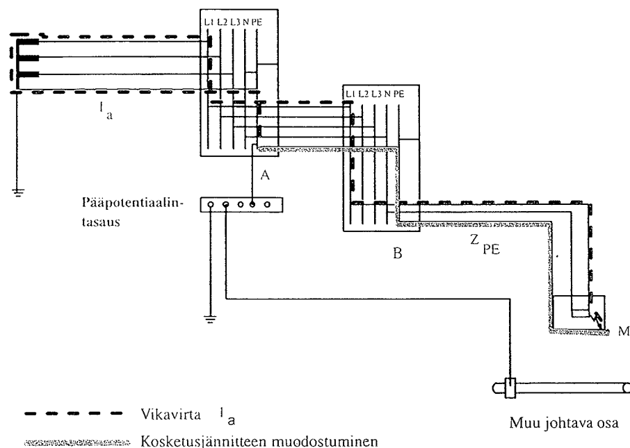
KUVA 41.11. Kosketusjännitteen muodostuminen vian aikana.
