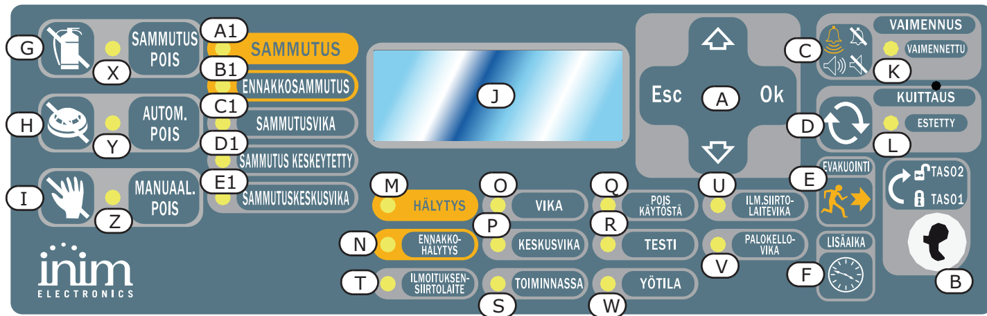
Kuva 6 - Ohjauspaneelin etuosa
