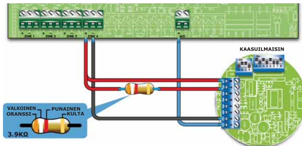
Kuva 15 - Kaasuilmaisimien yhdistäminen ilmaisulinjaan
