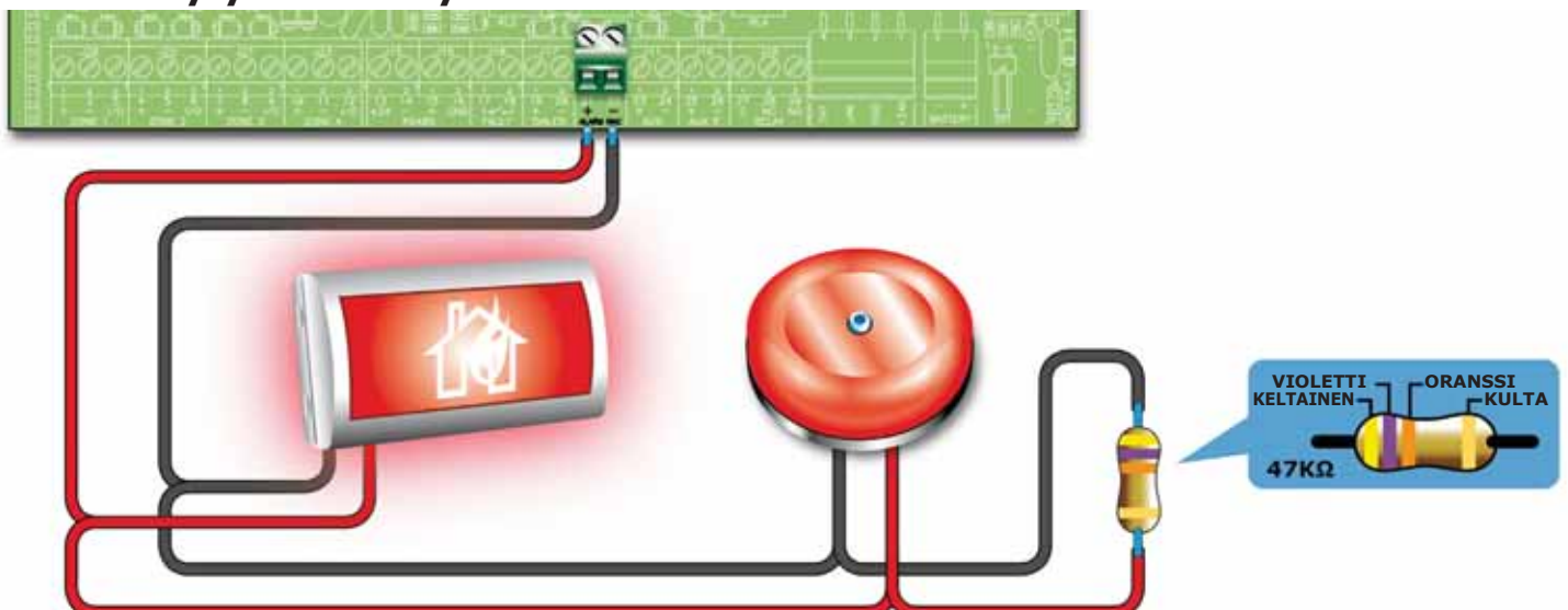
Kuva 26 - Hälytyslähdön yhdistäminen
