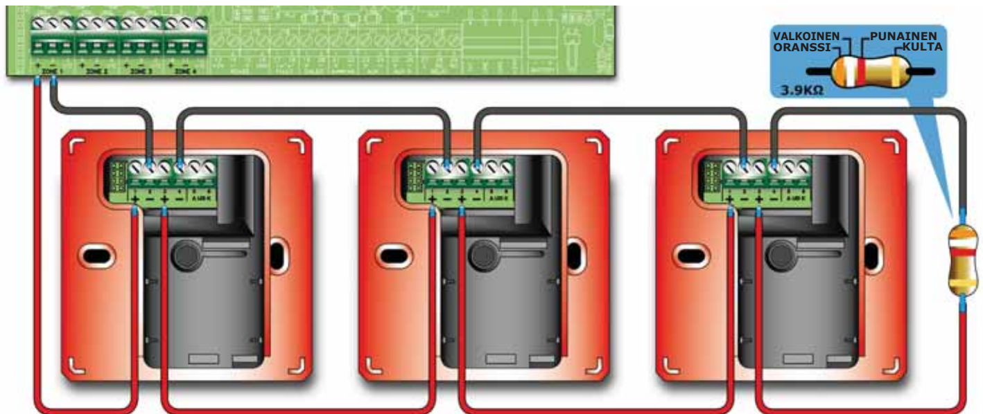
Kuva 13 - Iris-palopainikkeiden kytkentä
