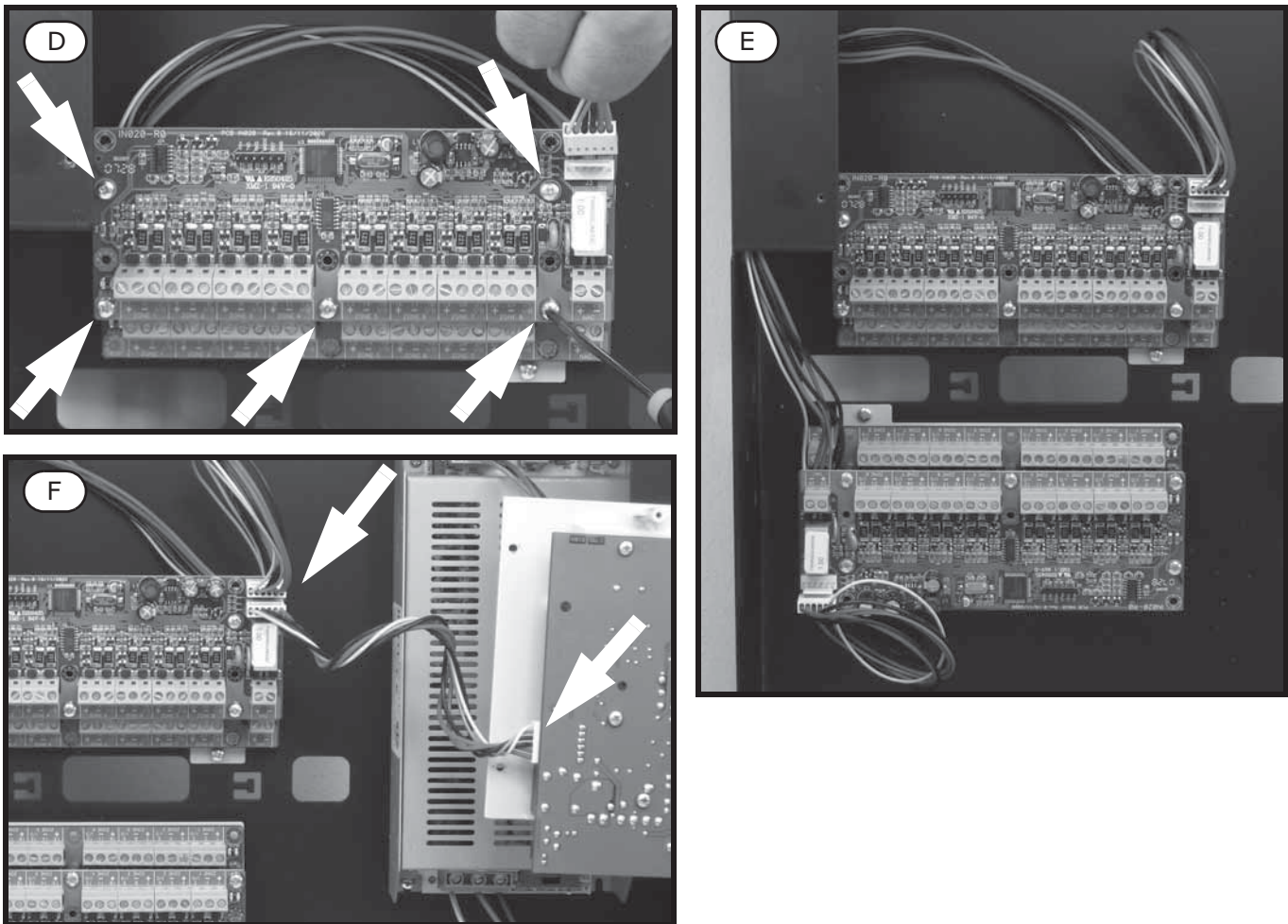
Kuva 10 - Laajennuskortin asennus - 2
