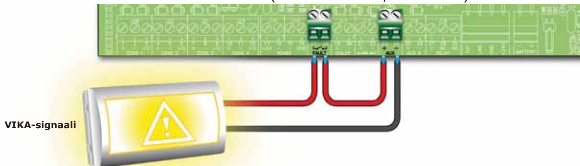
Kuva 25 - Vikamerkinantolähtöjen kytkeminen
