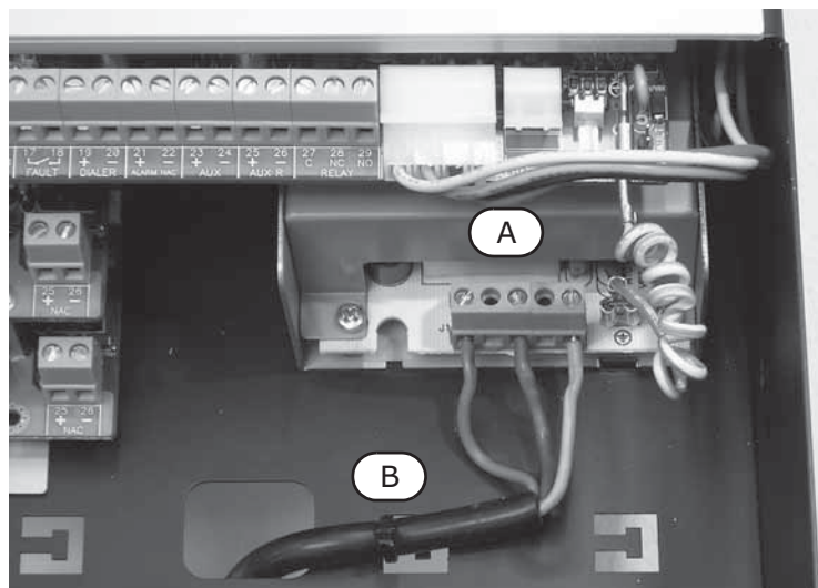
Kuva 30 - Verkkovirran kytkentä
