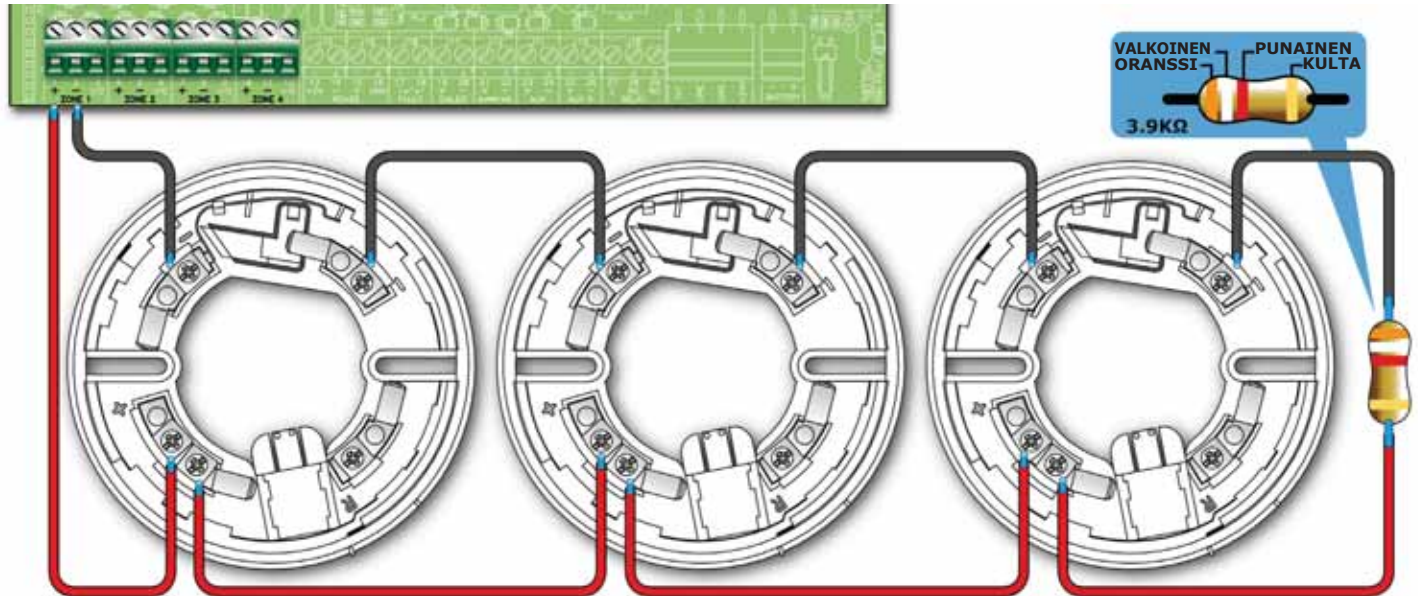
Kuva 12 - Iris-ilmaisimien kytkentä
