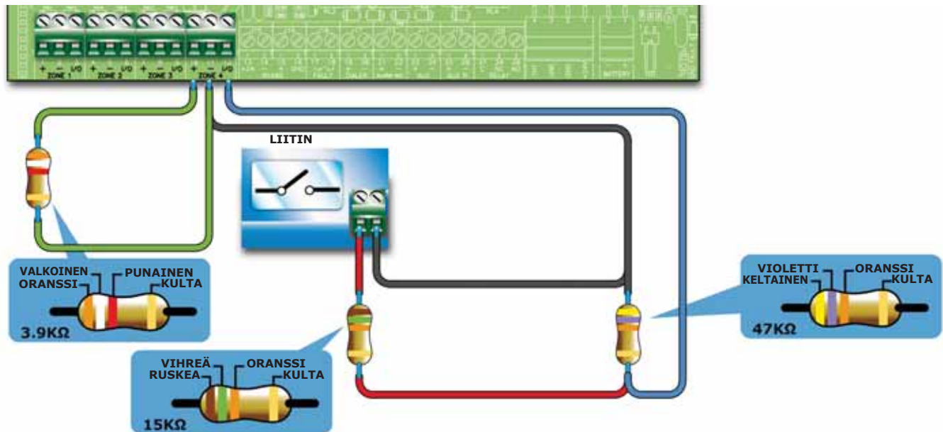
Kuva 18 - I/O-linjan kytkentä lähdeksi
