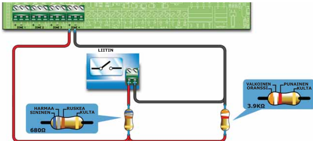
Kuva 16 - Yksikköjen kytkeminen ilmaisinjaan
