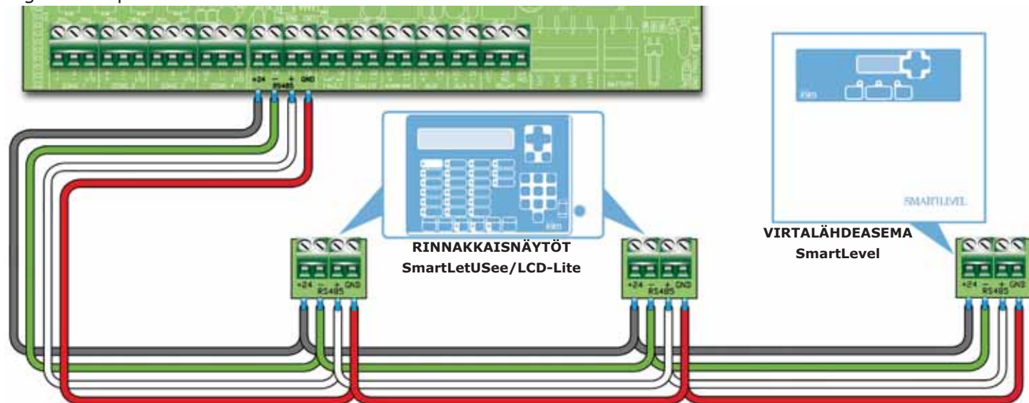
Kuva 22 - RS485-linjan yhdistäminen
