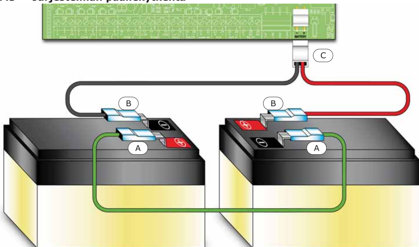
Kuva 34 - Akkujen kytkentä
