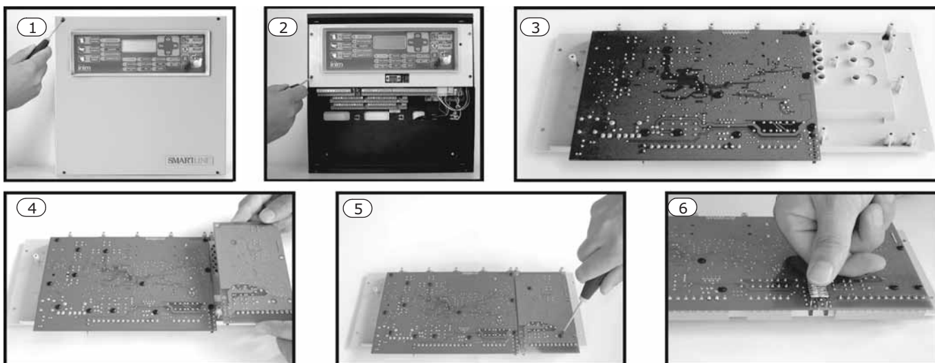
Kuva 11 - Sammutusmoduulin asennus
