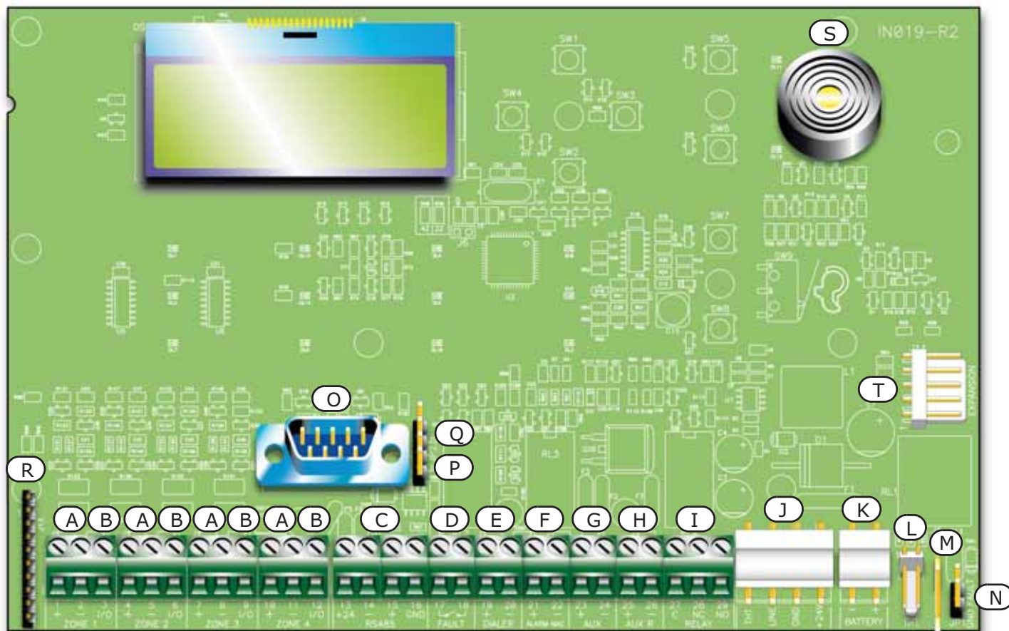
Kuva 5 - SmartLine-emolevy
