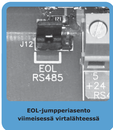
Kuva 24 - SmartLevel kortti - jumpperiasento
