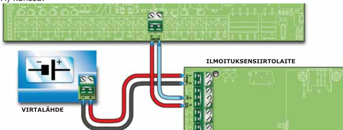
Kuva 20 - Ilmoituksensiirtolaitteen kytkentä
