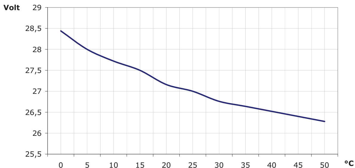
Kuva 32 - Jännite suhteessa akun lämpötilaan.
