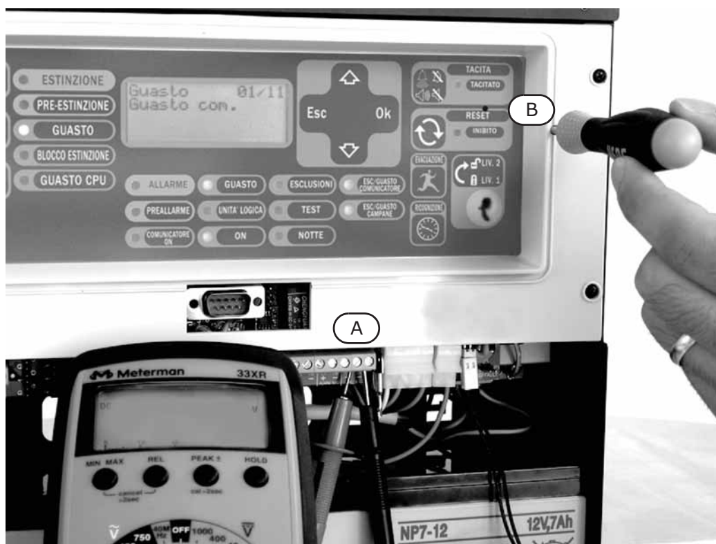
Kuva 33 - Jännitteen säätäminen
