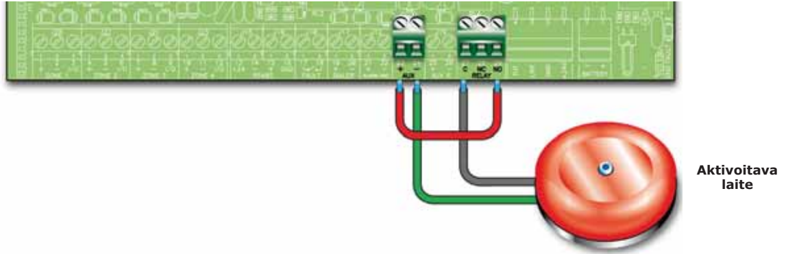
Kuva 28 - Relelähtöjen kytkentä
